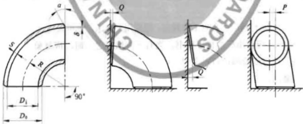
图 1 90° 弯头
