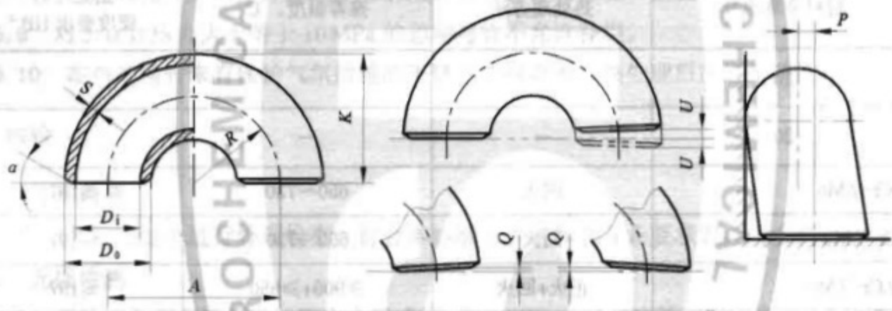
图 2 180° 急弯弯管
